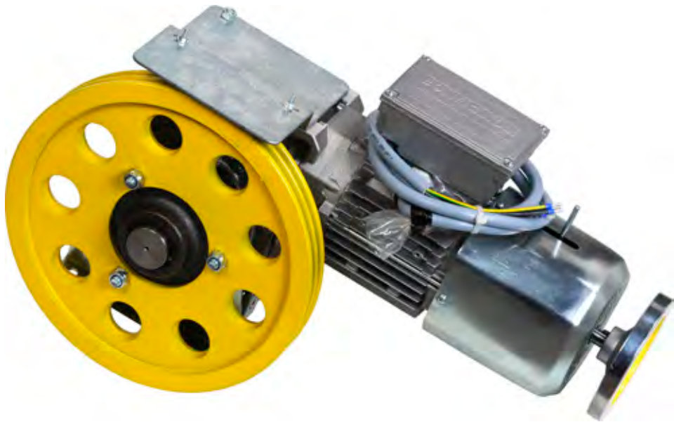
Triebwerk mit Nabe und Treibscheibe links
