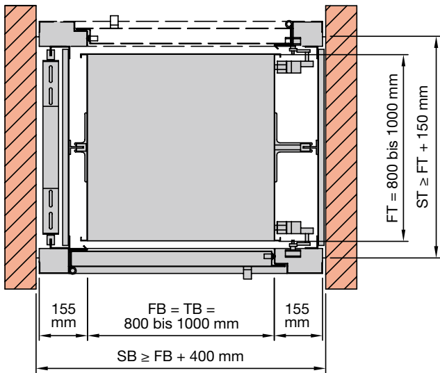
Triebwerksraumzugang
