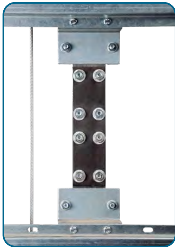
Verschraubte Gegenplatte
